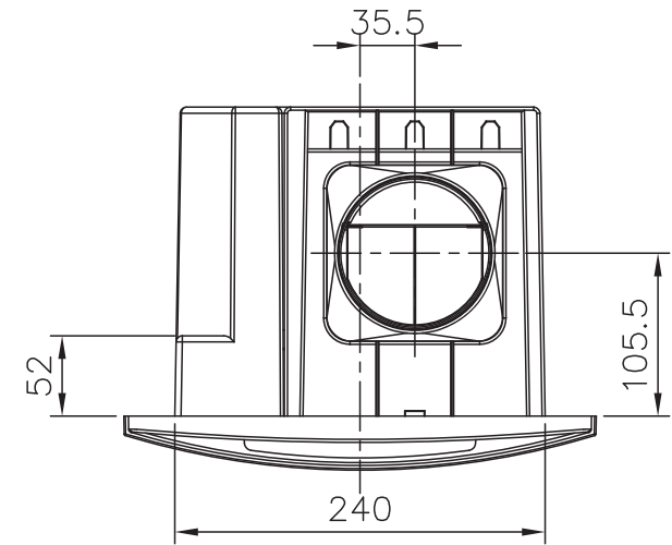
外觀尺寸圖 (單位 : mm)
