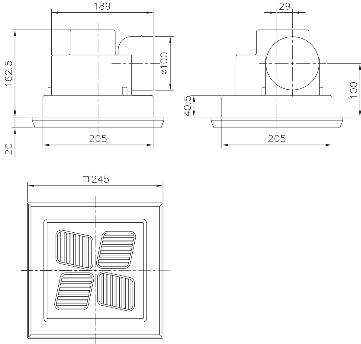
外觀尺寸圖 (單位 : mm)
